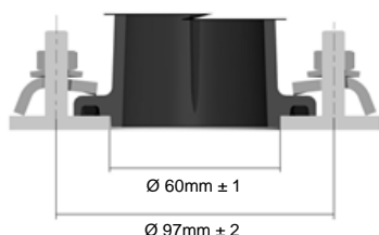
Instalación del DMCR
