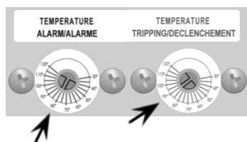
Interruptores de Termostato, Valores de Consigna
